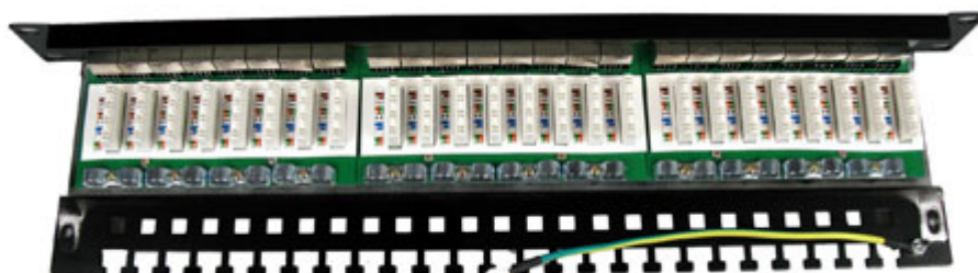
Horní pohled, konektory, zadní vyvazovací lišta a upínání kabeláže
